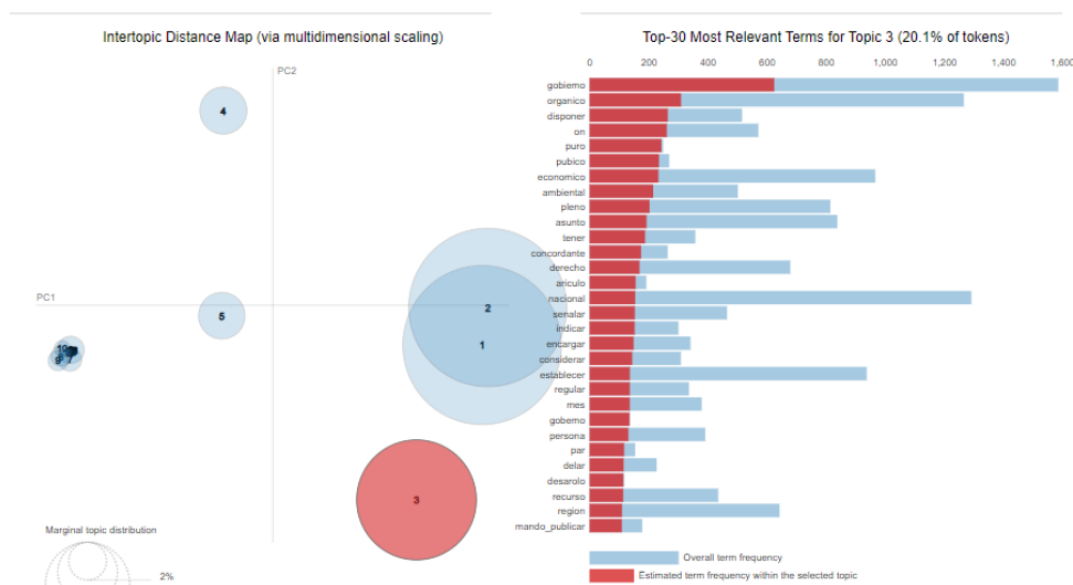
Figura 16. Tópico 3 del resultado del modelo LDA
