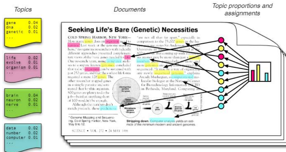
Figura 1. Intuición detrás de LDA.
