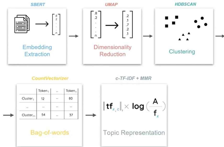
Figura 4. Pasos del modelo de tópicos BERTopic.
