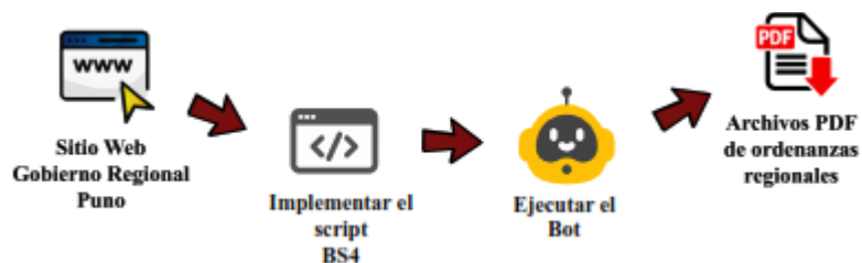
Figura 6. Pasos de extracción de datos mediante Web Scrapping .
