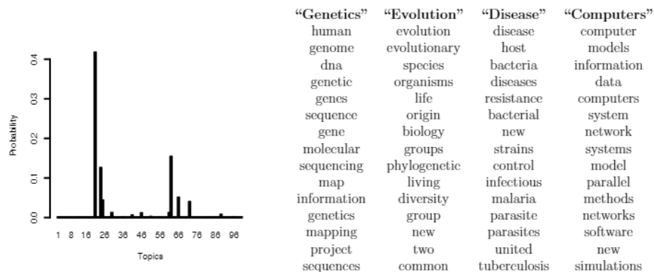
Figura 2. Inferencia real con LDA.
