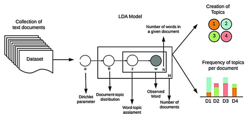
Figura 3. Modelado de tópicos basado en LDA
