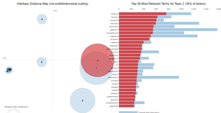
Figura 15. Tópico 2 del resultado del modelo LDA.
